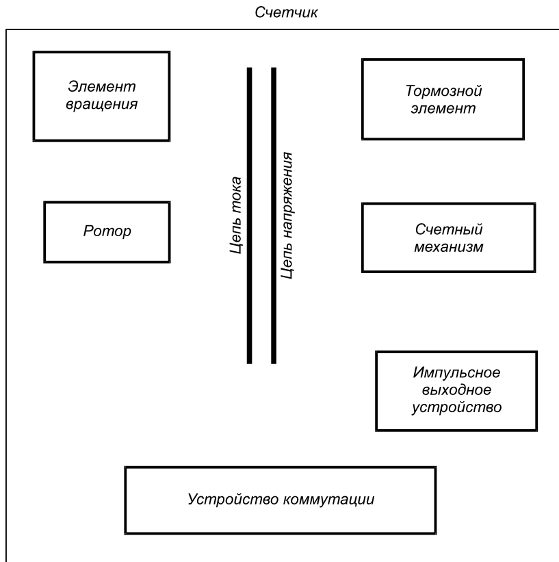
Рисунок С.1 — Структурная схема электромагнитного счетчика
